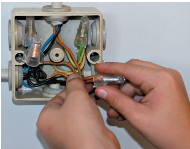
Herstellen einer Drehverbindung von Hand.
